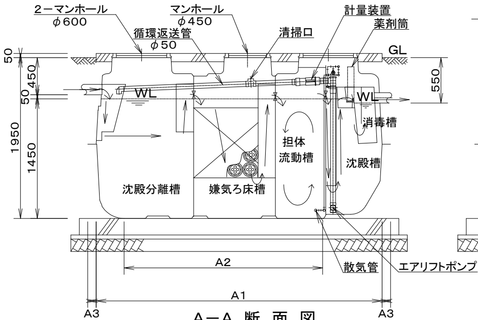
A-A断面図
