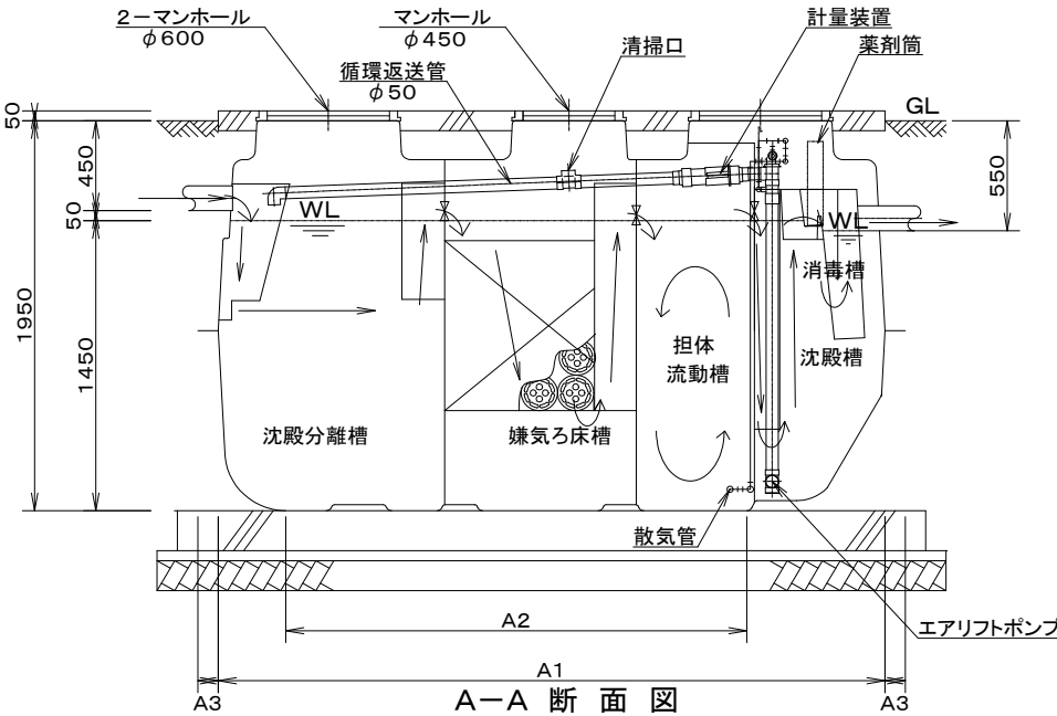
A-A断面図
