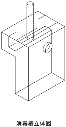
消毒槽立体図
