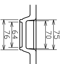
B-B断面
