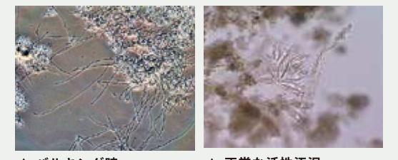
▲ バルキング時 ▲ 正常な活性汚泥
