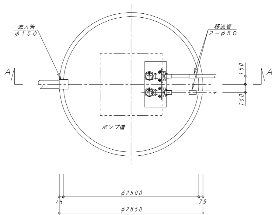
平面図 1:30
