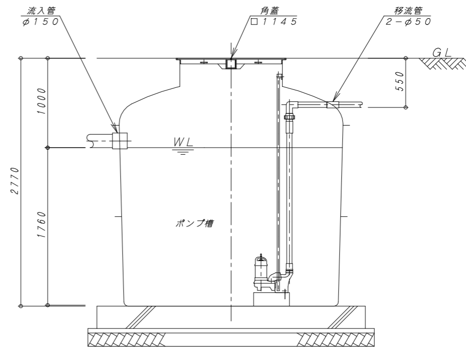
A-A 断面図 1:30
